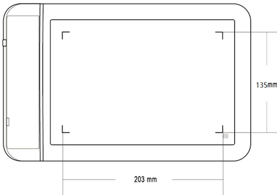
图 1-2. 感应区域
